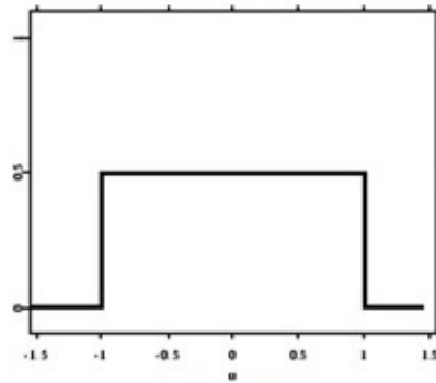
Uniforme
