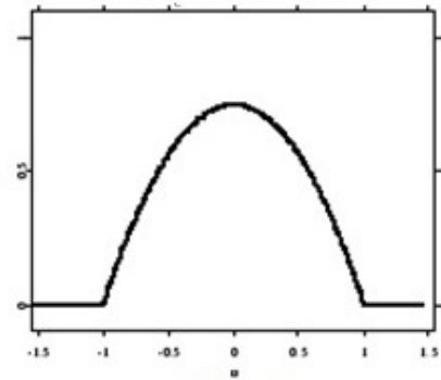
Epanechnikov
